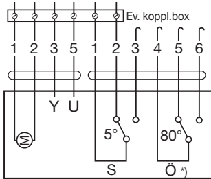
Ställdon
