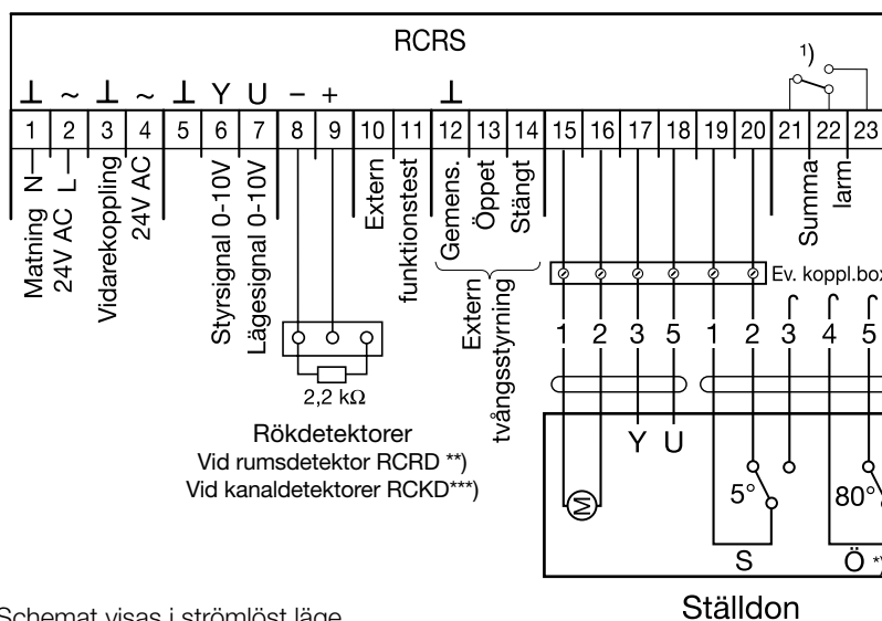
Schemat visas i strömlöst läge.
