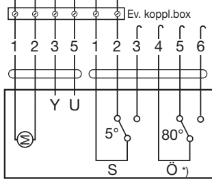
Ställdon
